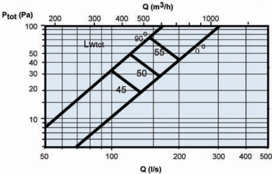
LDS.400 k=80,9 (l/s); 291 (m³/h)
